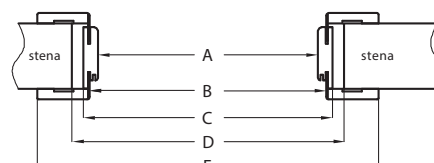
D - požadovaná šírka otvoru v mure
