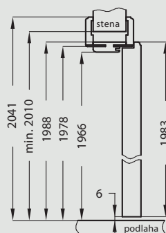
požadovaná výška otvoru v múre 2010 mm
