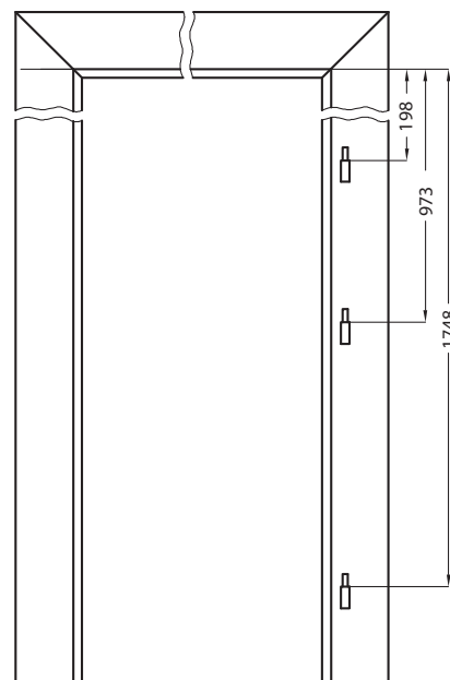
Vodorovný prierez
